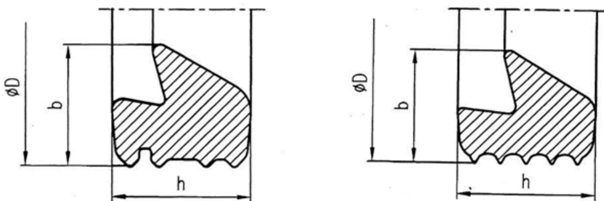
Рисунок 4 - Вид резинового уплотнительного одно лепесткового самоуплотняющегося типа
